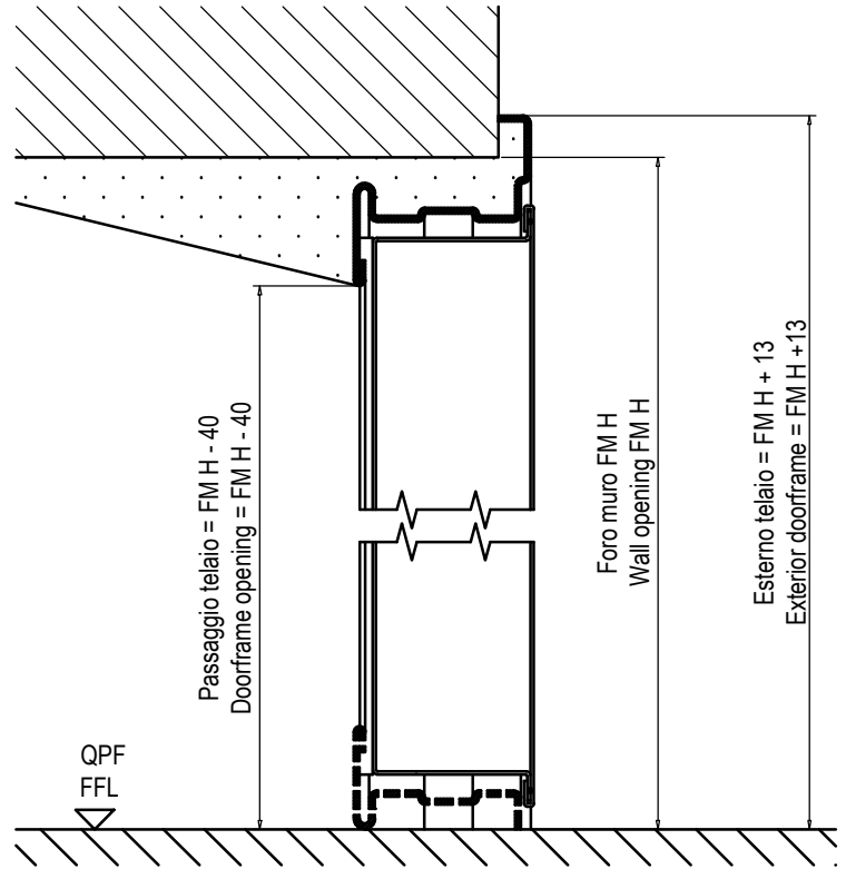
Sezione verticale Vertical cross section
